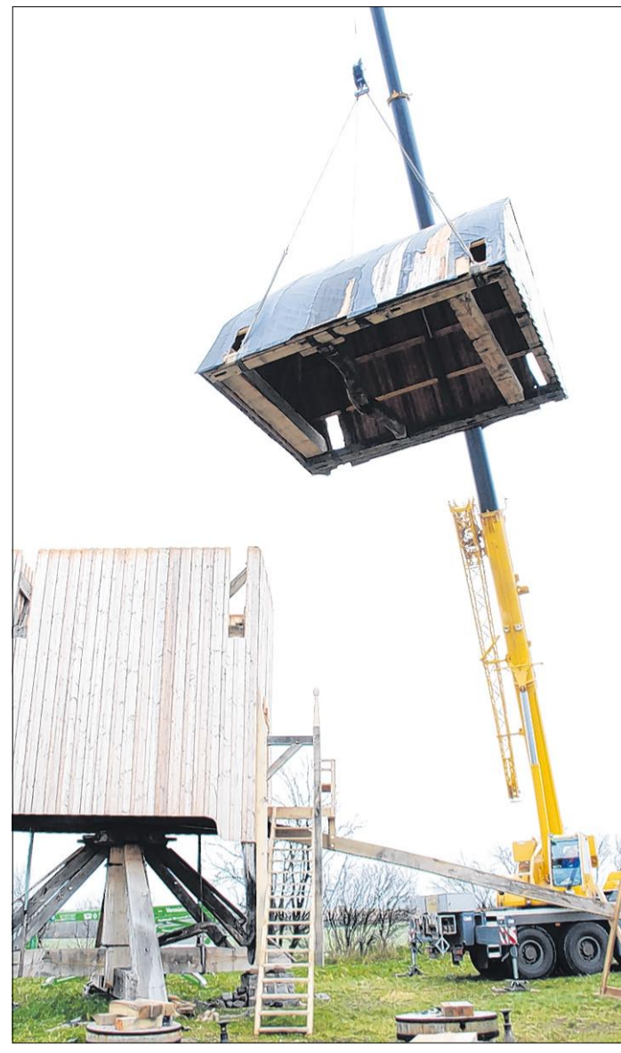
Für den Einbau der Rutenwelle wurde gestern die Dachhaube der Meseberger Windmühle abgenommen. Foto: Nico Maß
